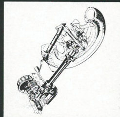
Rückfreier, wartungsarmer Kardanantrieb.
